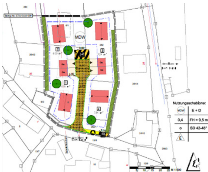
Auszug aus dem Planblatt des Bebauungsplanes „Baugebiet Nr. 1 Moosbach“ © Kartendarstellung: Bayerische Vermessungsverwaltung 2024
